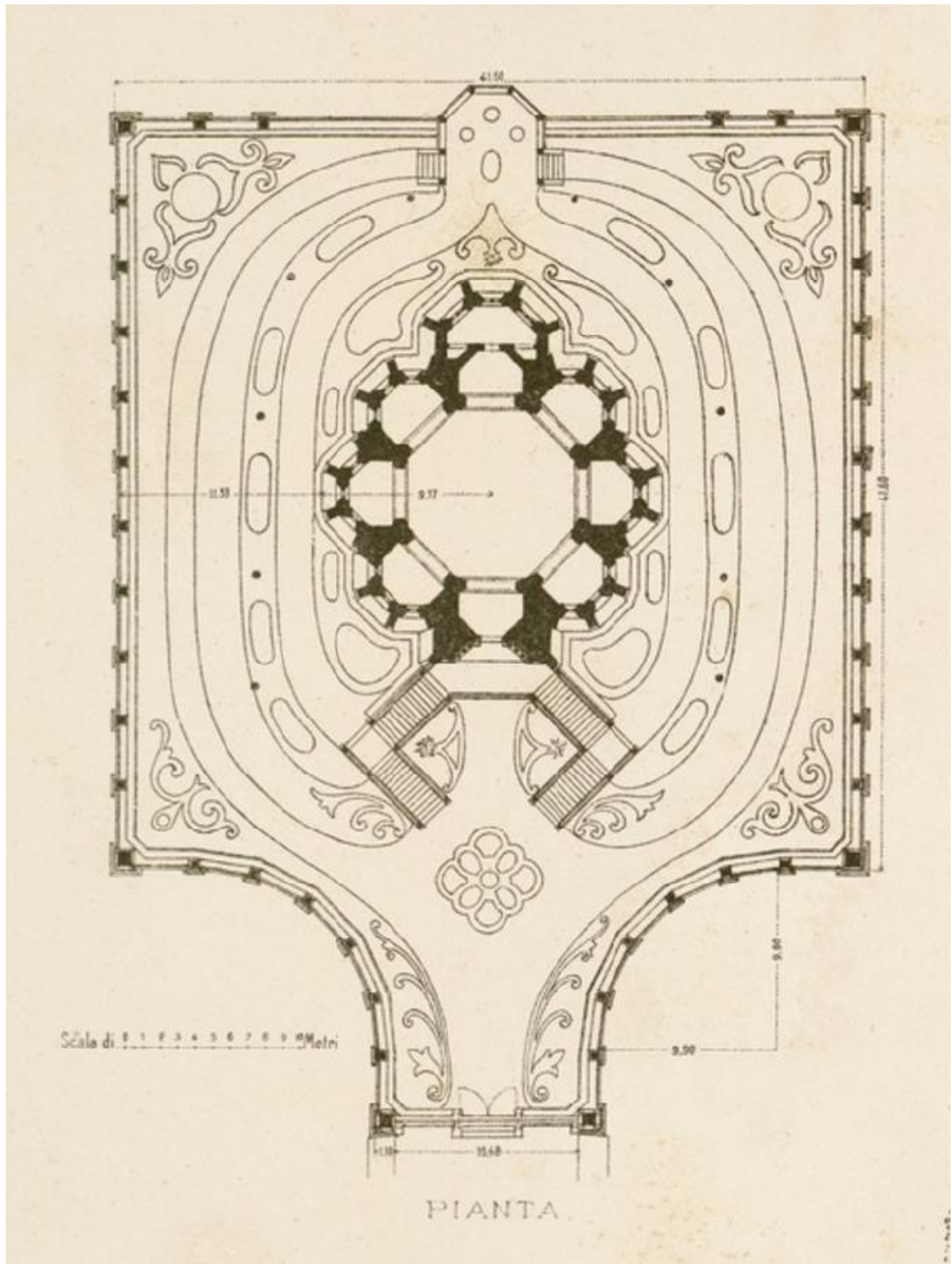
Cappella Sepolcrale della famiglia ducale Visconti di Modrone in Cassago (Bianza ). Pianta quotata
